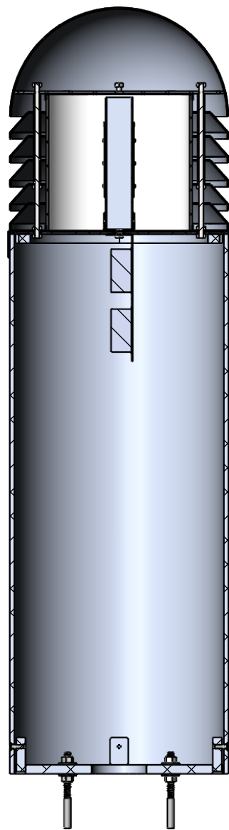
SECTION A-A
